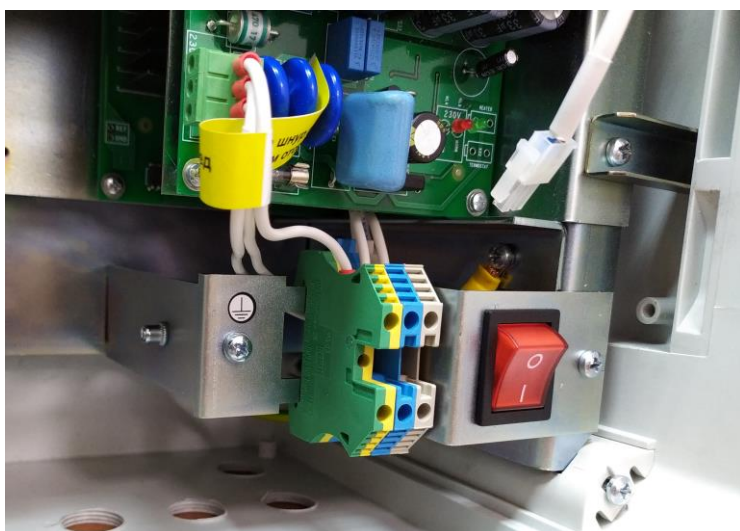
Рисунок 3.5.1 – Узел подключения питания.
