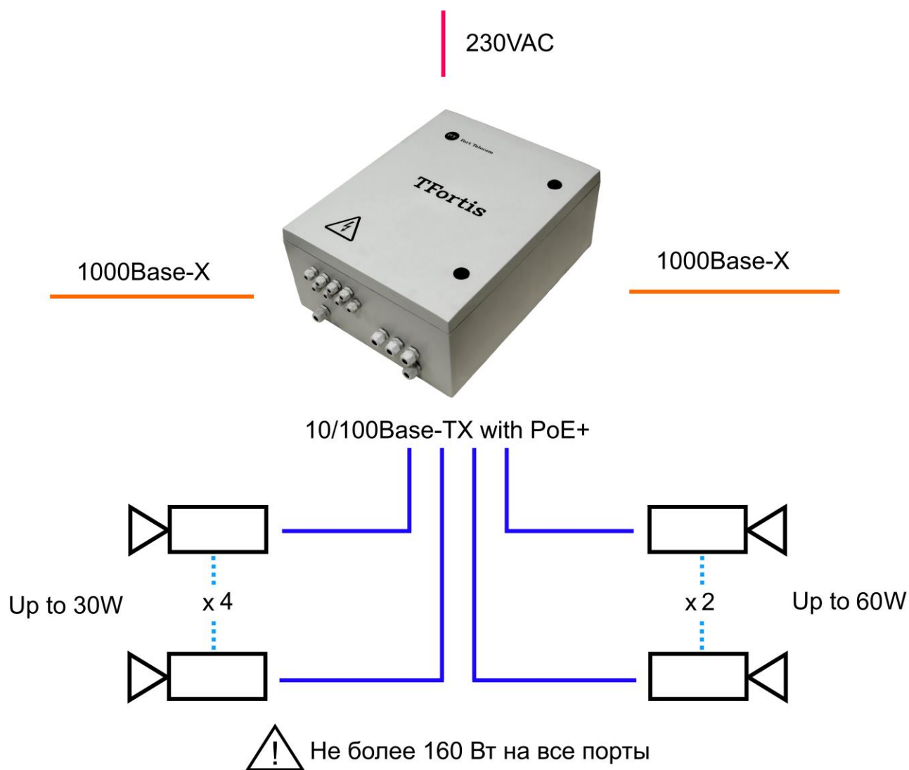
Рисунок 1 - Схема подключения PSW-2G6F+UPS-Box
