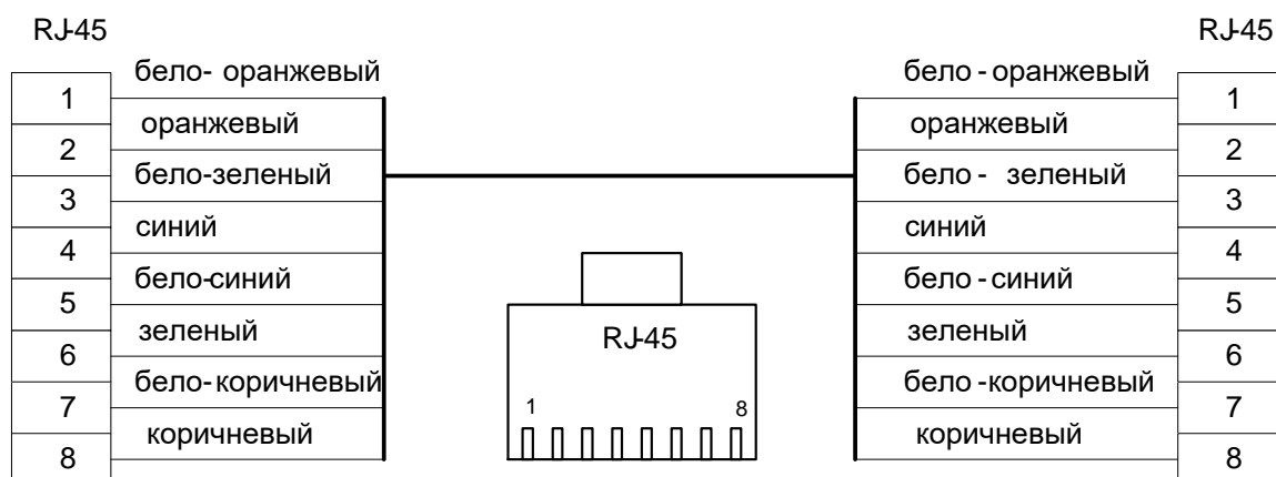
Рисунок 7.7 - Стандартная разделка кабеля.
