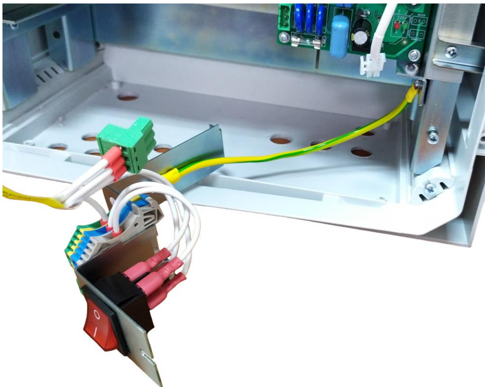
Рисунок 3.5.3 – Разъем питания 230 В отключен.
