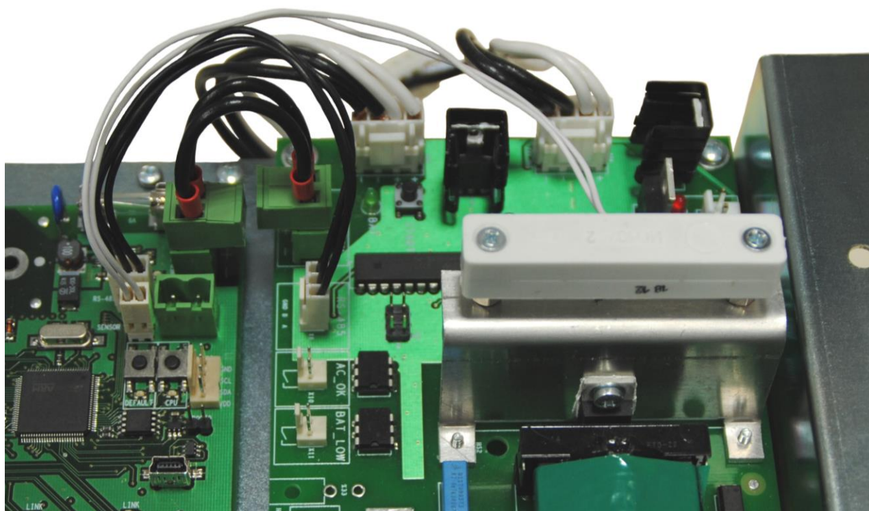
Рисунок 3.6.2 - Датчик вскрытия на корпусе коммутатора новая
