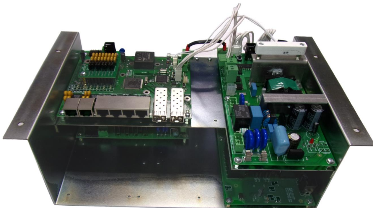
Рисунок 3.4.1 - Платы коммутатора и блоков питания
