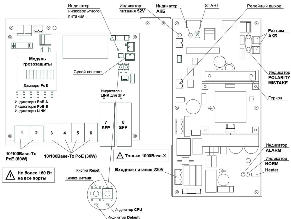
Рисунок 3.4.2 – Расположение элементов PSW-2G6F+UPS-Box
