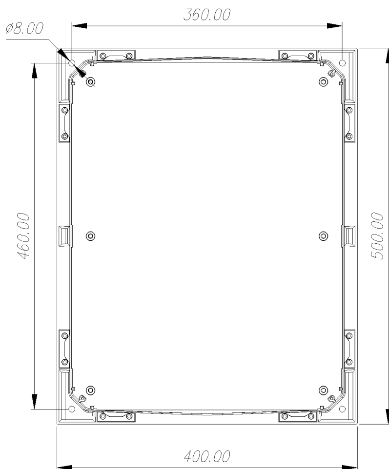
Рисунок 7.3 - Разметка крепления
